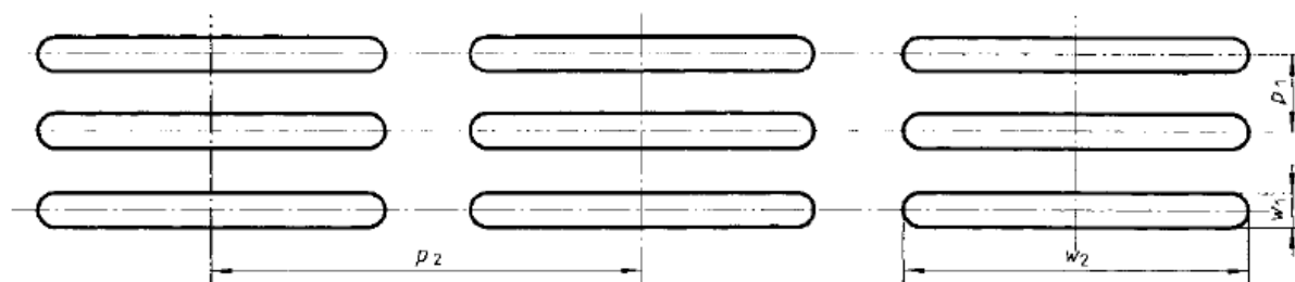
Slika 1. Otvori laboratorijskih sita sa dugačkim zaobljenim otvorima – linearni raspored (preuzeto iz ISO 5223:2013)
