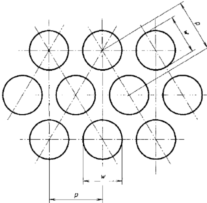
Slika 2. Otvori laboratorijskih sita sa okruglim otvorima – naizmenični raspored (centri otvora su raspoređeni u vrhove jednostranih trouglova) (preuzeto iz ISO 5223:2013)
